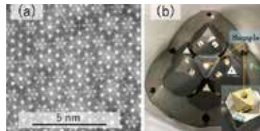
図(a)原子分解能での電子顕微鏡写真。点は原子です。 図(b)高圧発生装置の内部写真。数百トンの荷重を加えて、10万気圧以上の圧力を発生させます。
