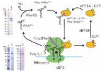
必要な分子だけでできた翻訳反応系
