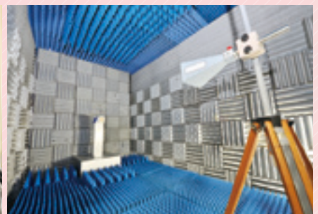
手作り電波暗室
